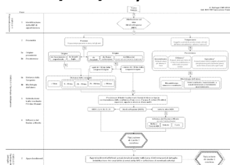
Figura 1.2 Tipologia per l'attribuzione di tratti fluviali ad un «tipo» ai sensi della Direttiva 2000/60/CE, Sistema B. Diagramma di flusso per il Livello 2
